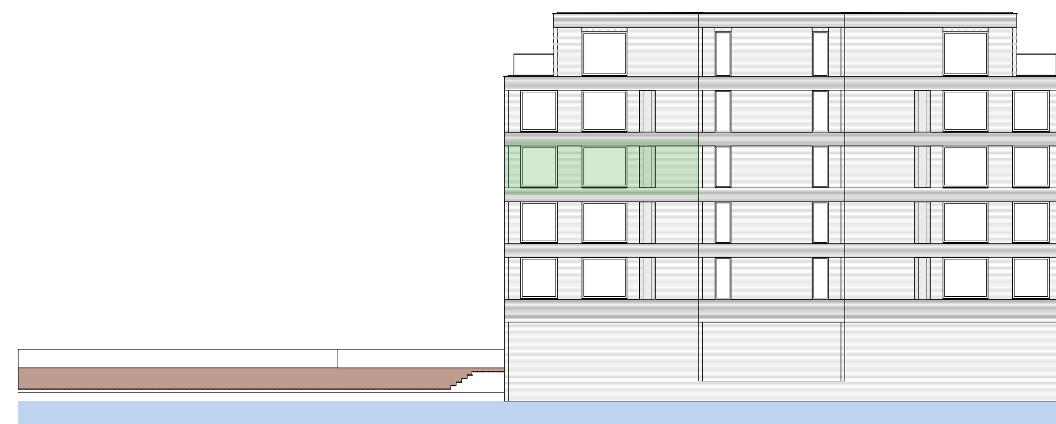
gevelaanzicht Noord-Oost 1: 200
