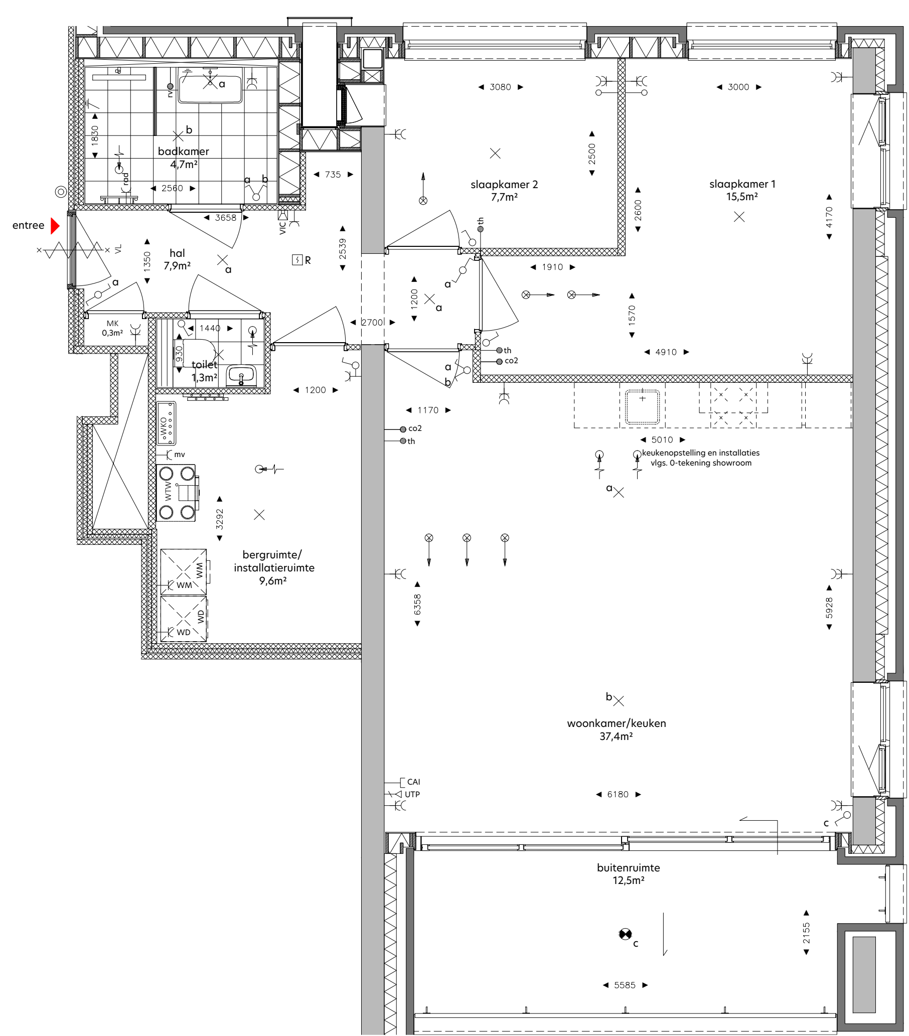
plattegrond 1: 50
