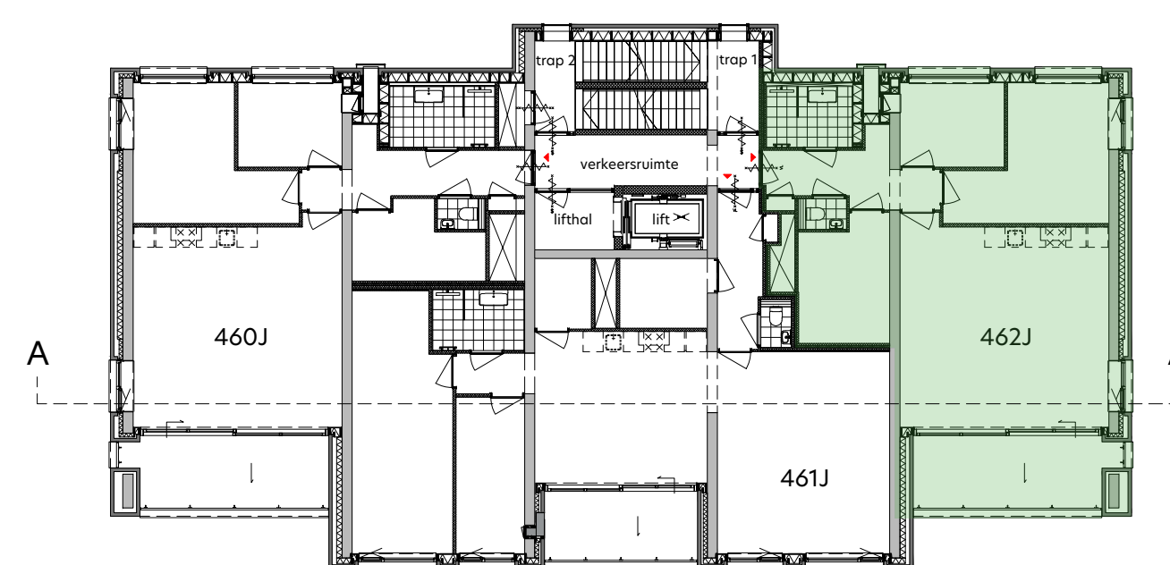
overzicht derde verdieping 1: 200
