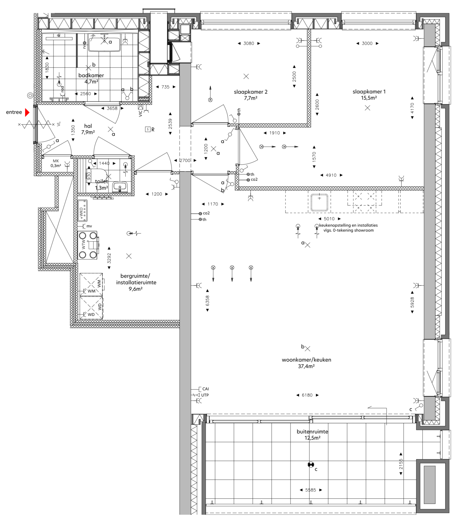
plattegrond 1: 50
