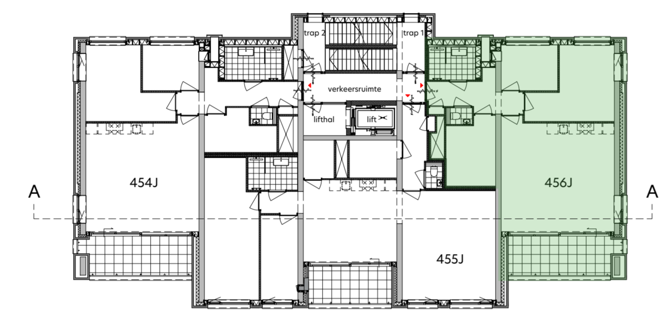
overzicht eerste verdieping 1: 200
