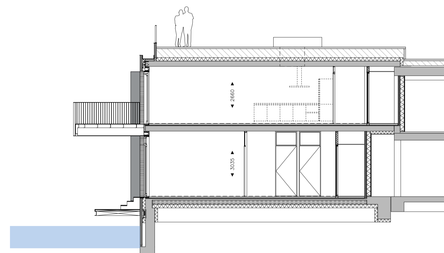
doorsnede A-A 1: 100
