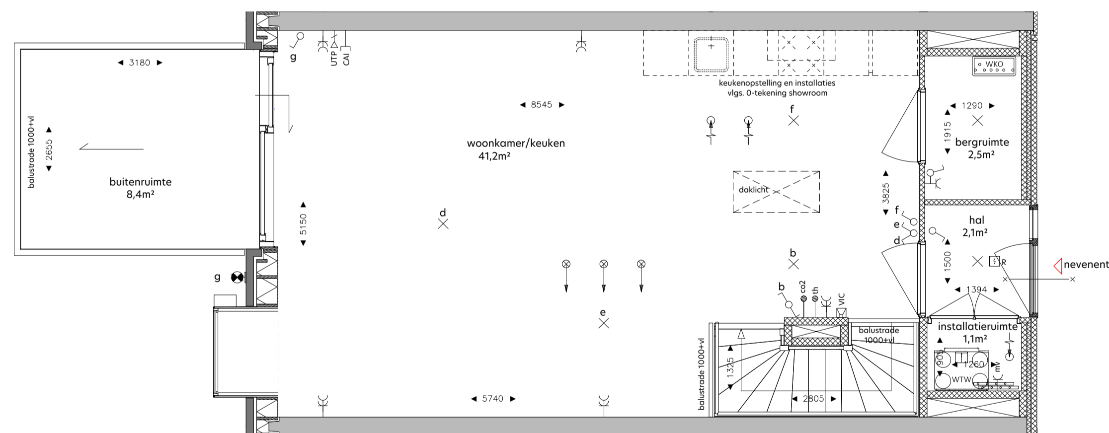
plattegrond eerste verdieping 1: 50
