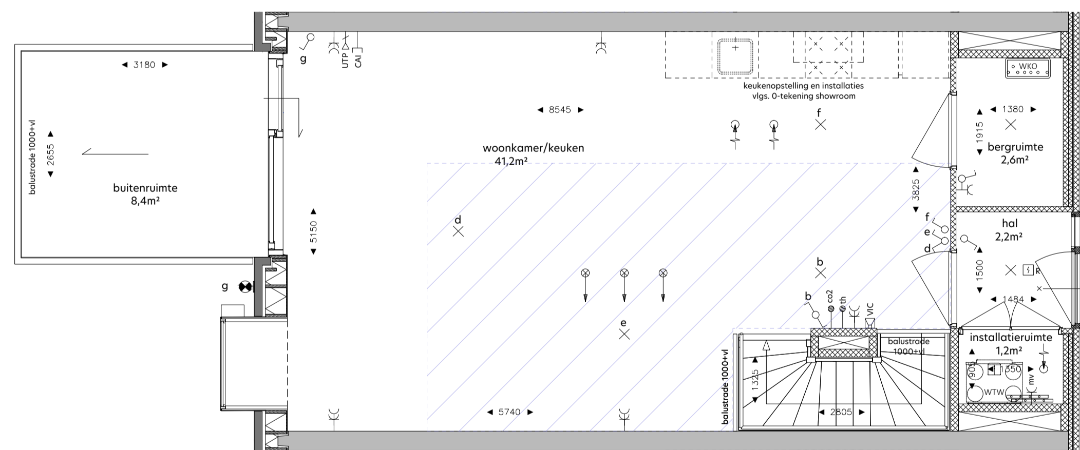
plattegrond eerste verdieping 1: 50
