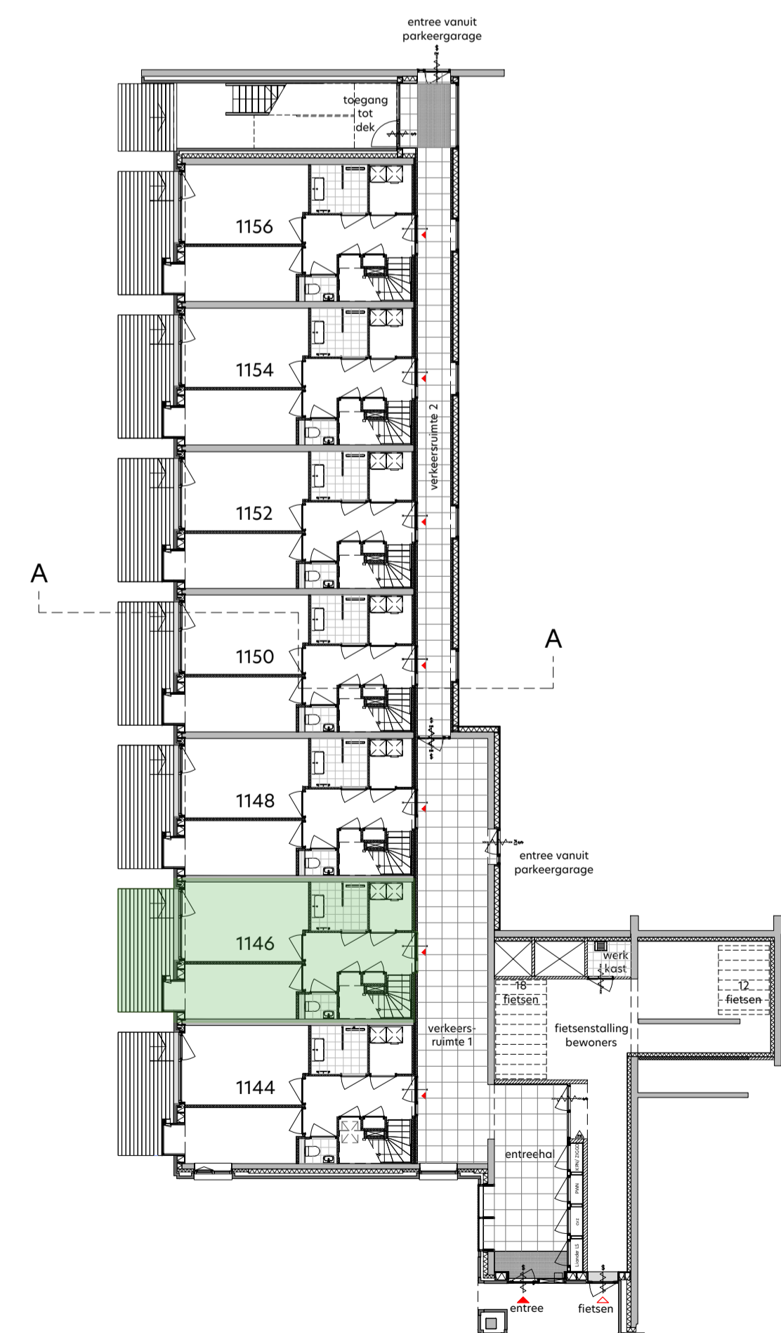
overzicht begane grond 1: 200
