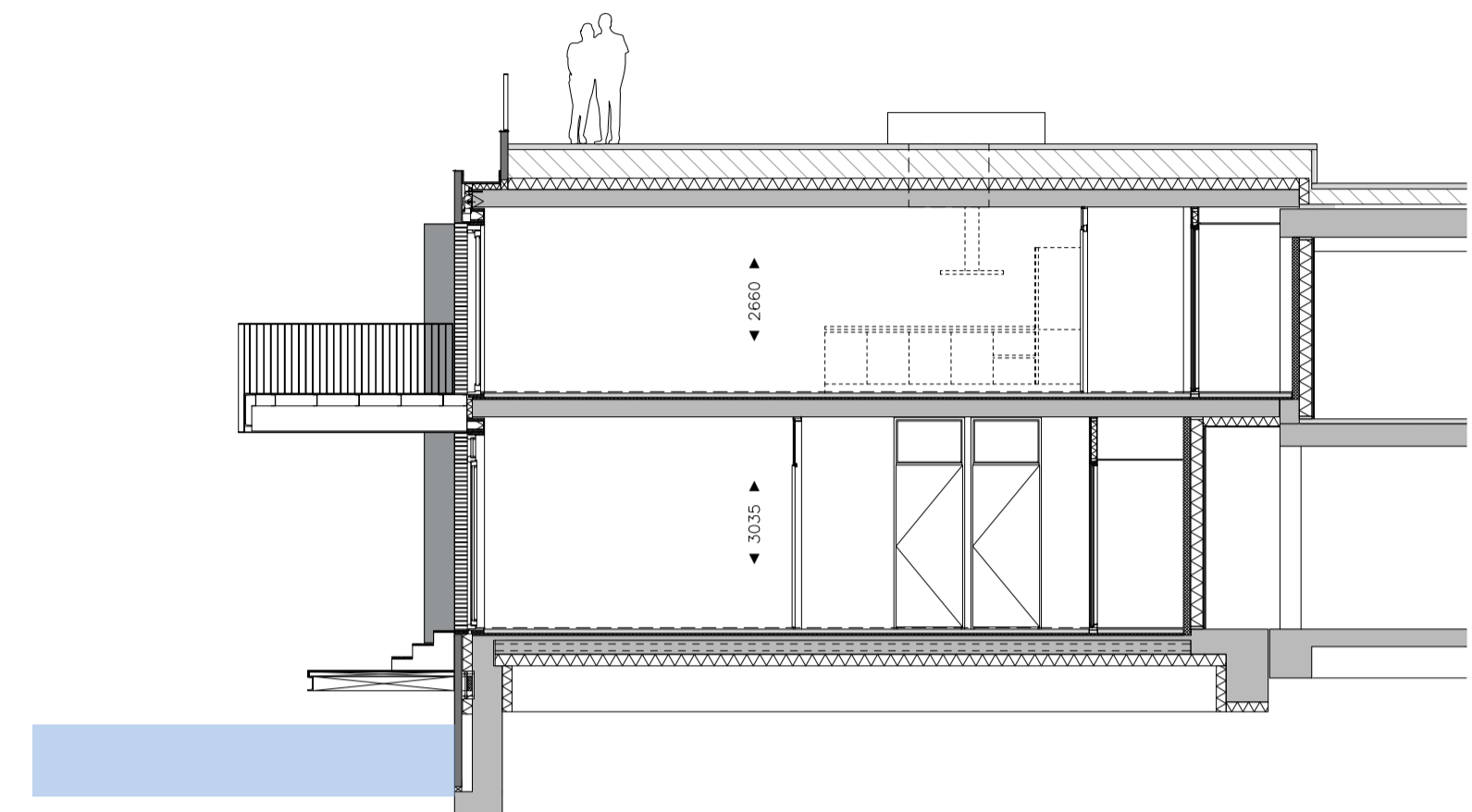
doorsnede A-A 1: 100
