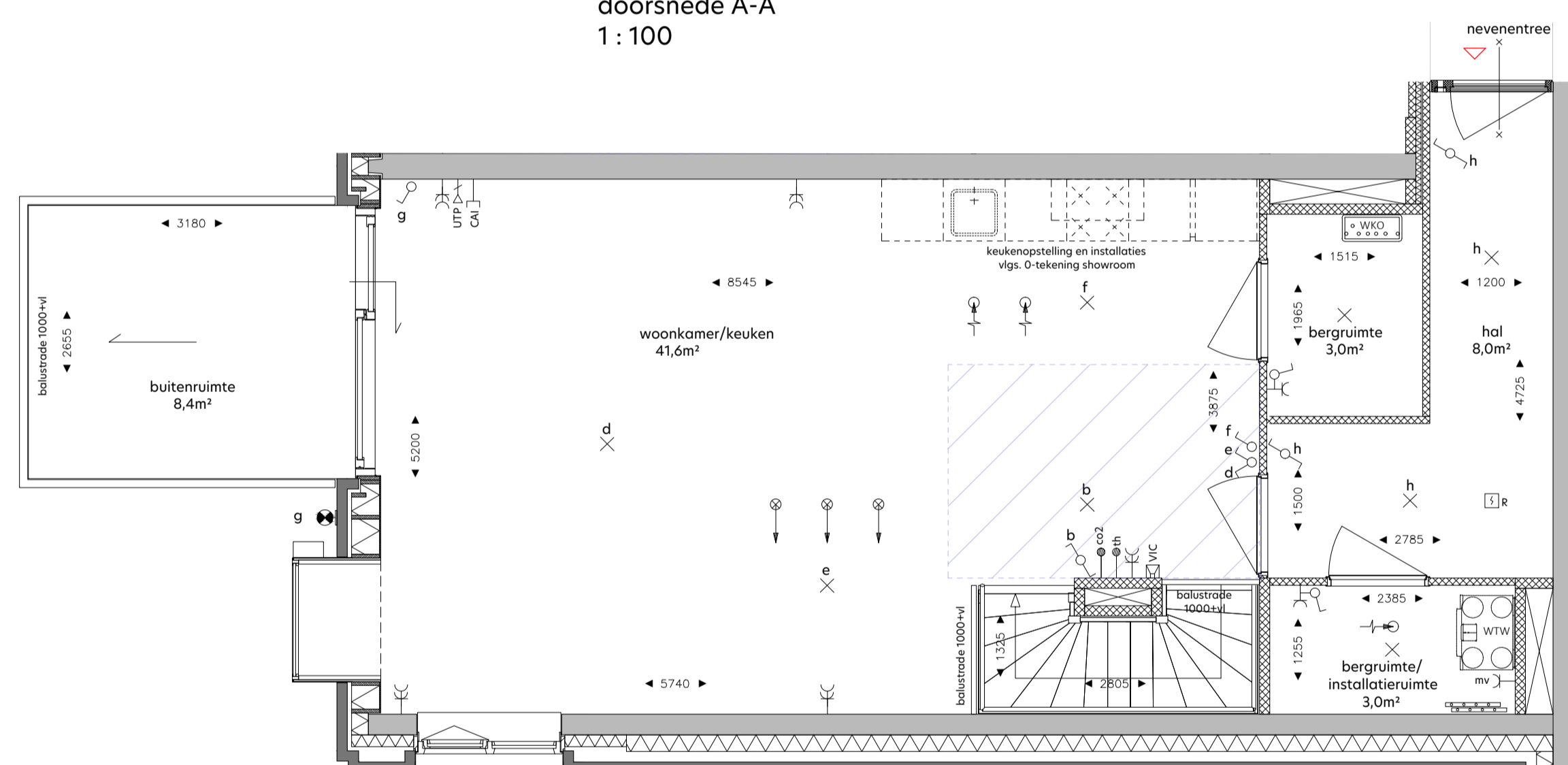
plattegrond eerste verdieping 1: 50
