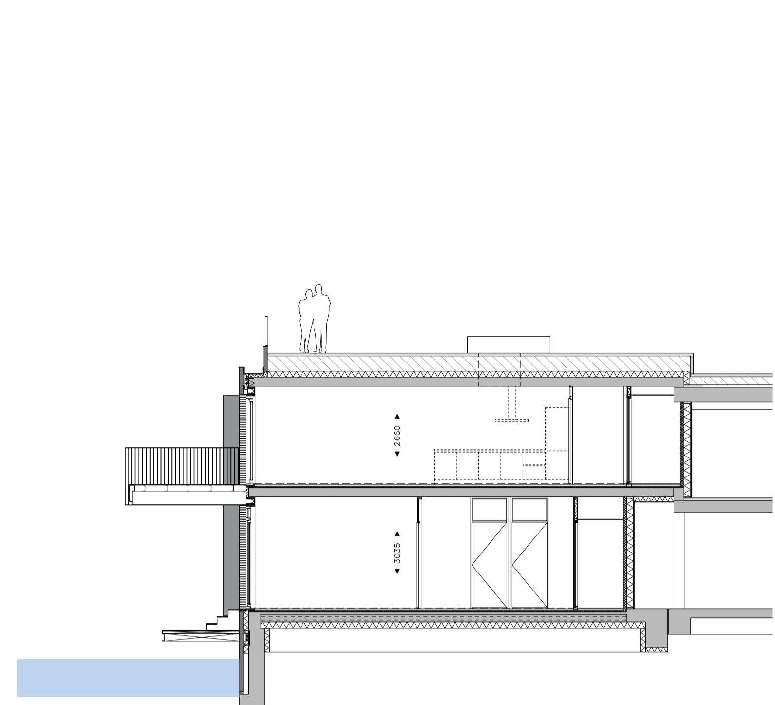
doorsnede A-A 1: 100
